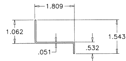
42A LOUVER FRAME (1-3/4")
