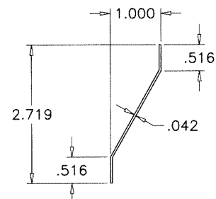
43 LOUVER BLADE (1")
